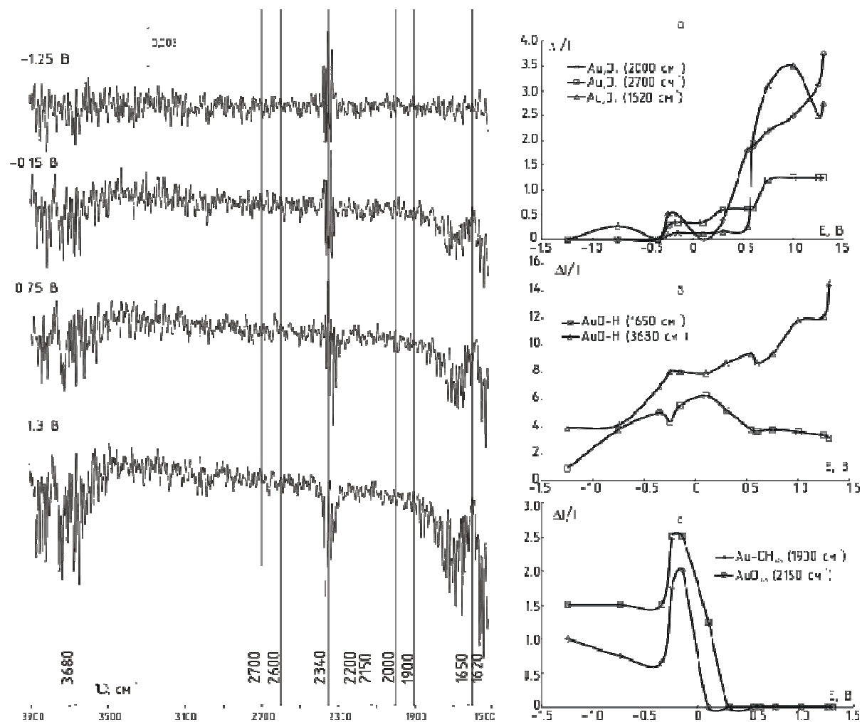
Рис. 4. Результаты in situ FTIR-спектроскопии системы \text{Au(OH)}^- при 298\text{ К}
