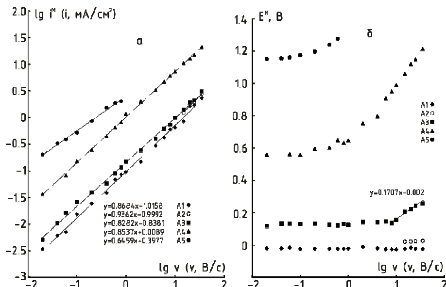
Рис. 2. Зависимость логарифма тока пика (а) и потенциала пика (б) от скорости сканирования при C_{\text{OH}^-} = 0,1 \text{ M}
