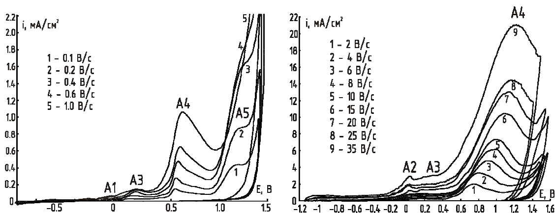
Рис. 1. Циклические вольтамперограммы Au-электрода в растворе 0,1 М NaOH при различных скоростях сканирования потенциала
