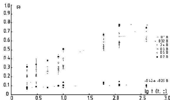
Рис. 5. Накопление различных форм кислорода на Au в 0,1 М NaOH
