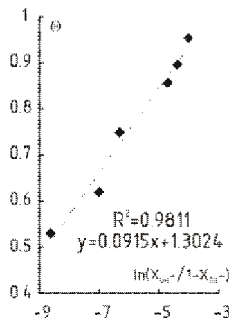
Рис. 6. Стационарная изотерма адсорбции кислорода в системе \text{Au}|\text{OH}^- при E = 0,60 В
