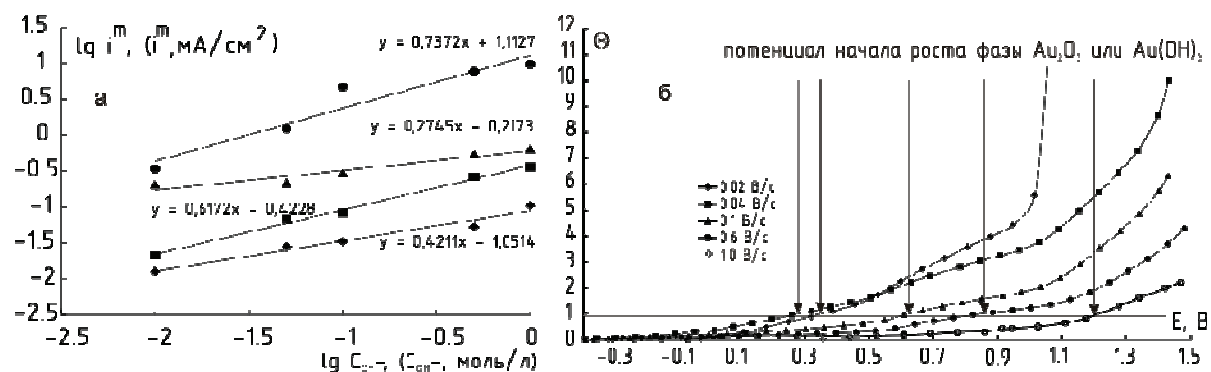
Рис. 3. (а) Зависимость тока от концентрации гидроксид-ионов при v = 0,06\text{ В/с} ; (б) Влияние потенциала на степень заполнения поверхности золота кислородом при C_{\text{OH}^-} = 0,1\text{ М}
